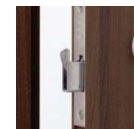
B81型
